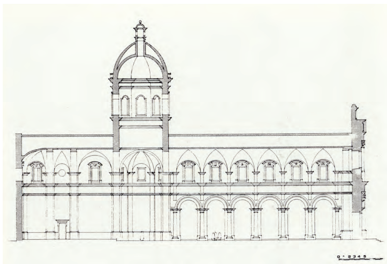
17 Sezione della Basilica
