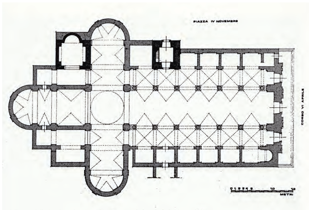
16 Pianta della basilica, progetto dell'arch. Angelo Italia, a. 1699.
